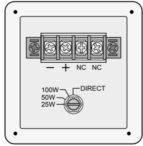
Exemple PAB-6WP/WS : puissance nominale réglée = 25 W Esempio PAB-6WP/WS: potenza nominale impostata = 25 W
