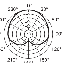
1 Diagrama polar a 1 kHz Wykres biegunowy przy 1 kHz
